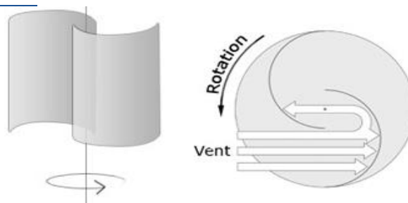
شکل شماره «۷۳»: انواع توربین‌های بادی با محور چرخش عمودی در پلان و نما
