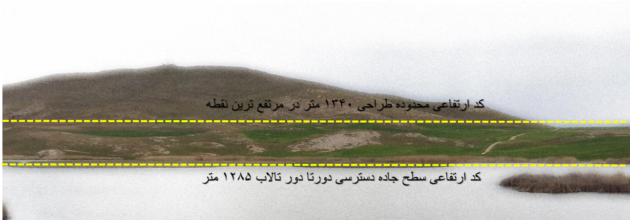
شکل شماره «۱۱»: وضعیت شیب محدوده نقطه D در دید مستقیم از مقابل ساختمان پرنده نگری موجود (اختلاف ارتفاع حدود ۳۵ متر)
