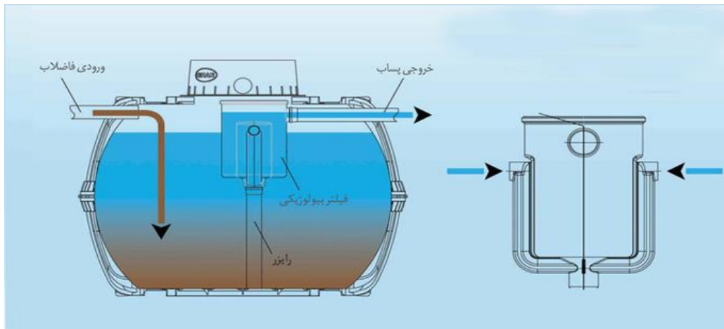
شکل شماره «۷۸»: سیستم کارکرد سپتیک تانک دارای فیلتر بی‌هوازی و نحوه تصفیه بیولوژیک آن.
