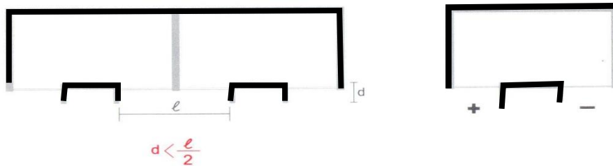
شکل شماره «۳۰»: عمق تیغه‌های عمودی لام در کنار پنجره‌ها جهت ایجاد کوران در داخل اتاق
