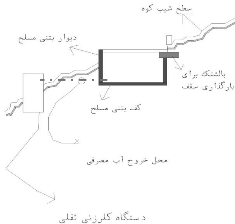
طرح شماتیک از جایگذاری مخزن - سطوح آبگیر و دستگاه کلر زنی نسبت به هم
