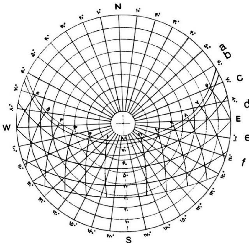
شکل شماره «۲۷»: موقعیت و زوایای تابش خورشید در عرض جغرافیایی ۳۷ درجه .
