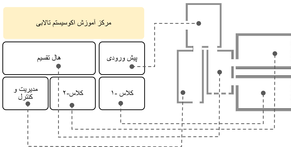
شکل شماره «۹۳»: پلان شماتیک مرکز آموزش اکوسیستم تالابی - سایت A - پلان نشان دهنده فرم نهایی نیست
