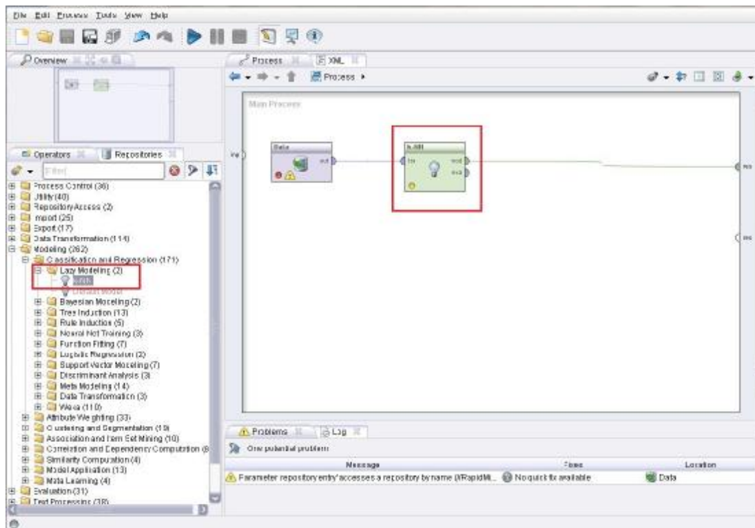
شکل 3-1: انتخاب الگوریتم KNN و داده‌ها
