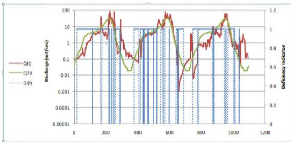
شکل 3-6: تغییرات سری‌های زمانی دبی، دبی‌های 70% و شاخص DI در ایستگاه ونیار
