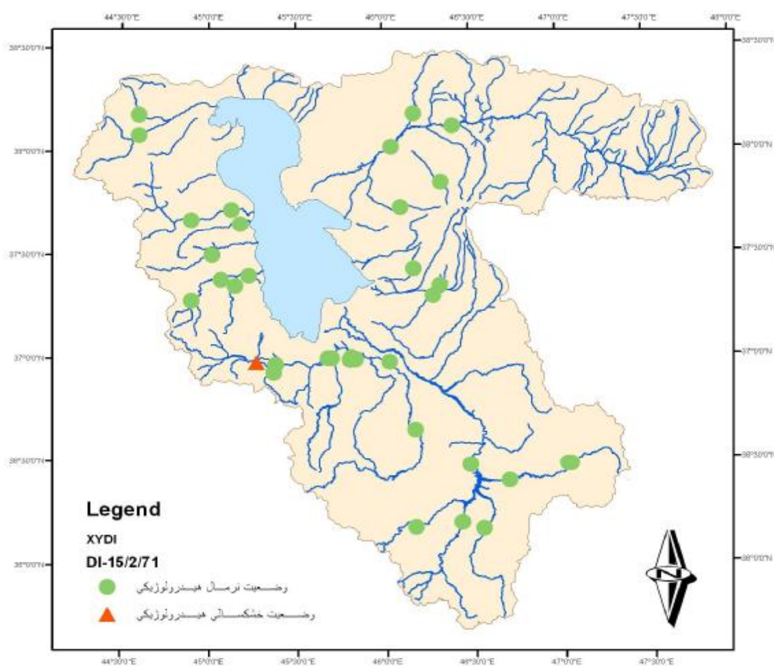
شکل 3-7: وضعیت هیدرولوژیکی خشکسالی در حوضه دریاچه ارومیه در تاریخ 1371/2/15
