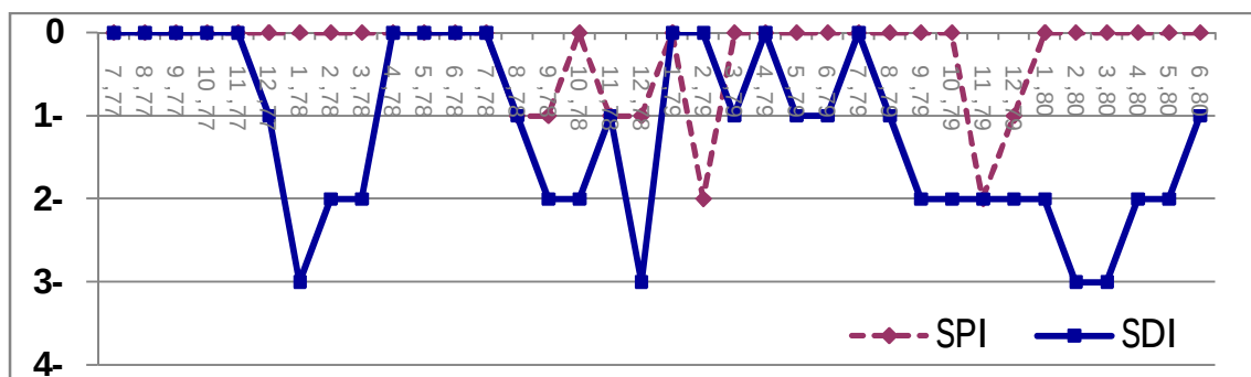
شکل 3-15: نمودار مقایسه شاخص های SPI و SDI برای ایستگاه های نقده طی سال های آبی 1377-78 تا 1379-80
