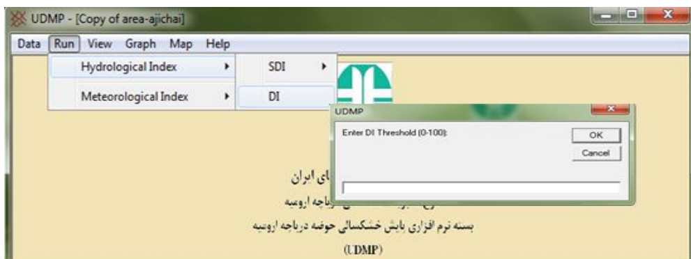
شکل 3-5: محاسبه شاخص DI در مدل UDMP و معرفی آستانه دبی
