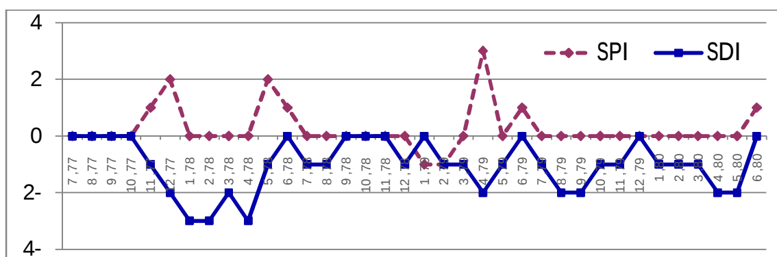
شکل 3-14: نمودار مقایسه شاخص‌های SPI و SDI برای ایستگاه‌های سنه طی سال‌های آبی 1377-78 تا 1379-80
