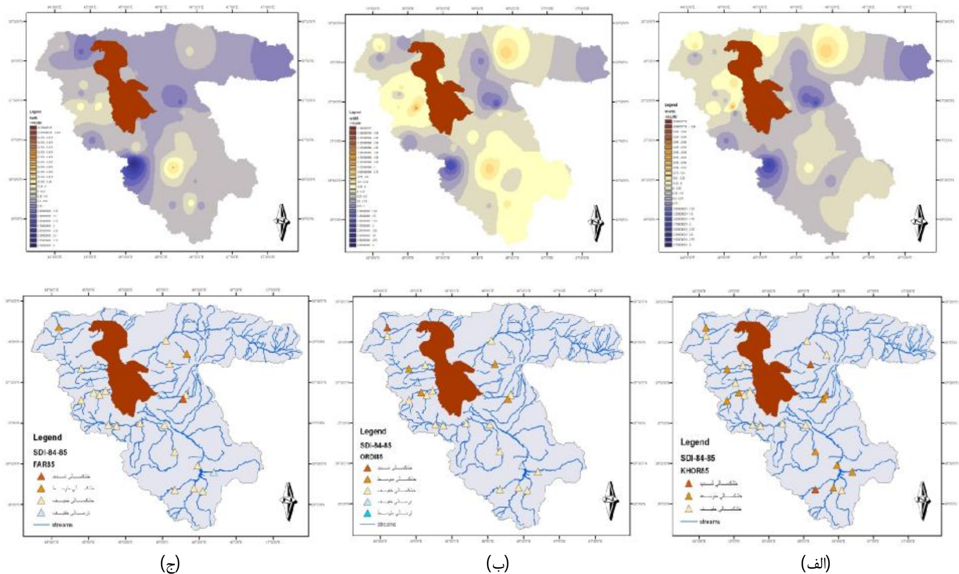
شکل 3-18: مقایسه توزیع مکانی شاخص SPI و شاخص SDI در حوضه دریاچه ارومیه در سال آبی 84-85 در ماه‌های الف) فروردین، ب) اردیبهشت، ج) خرداد.
