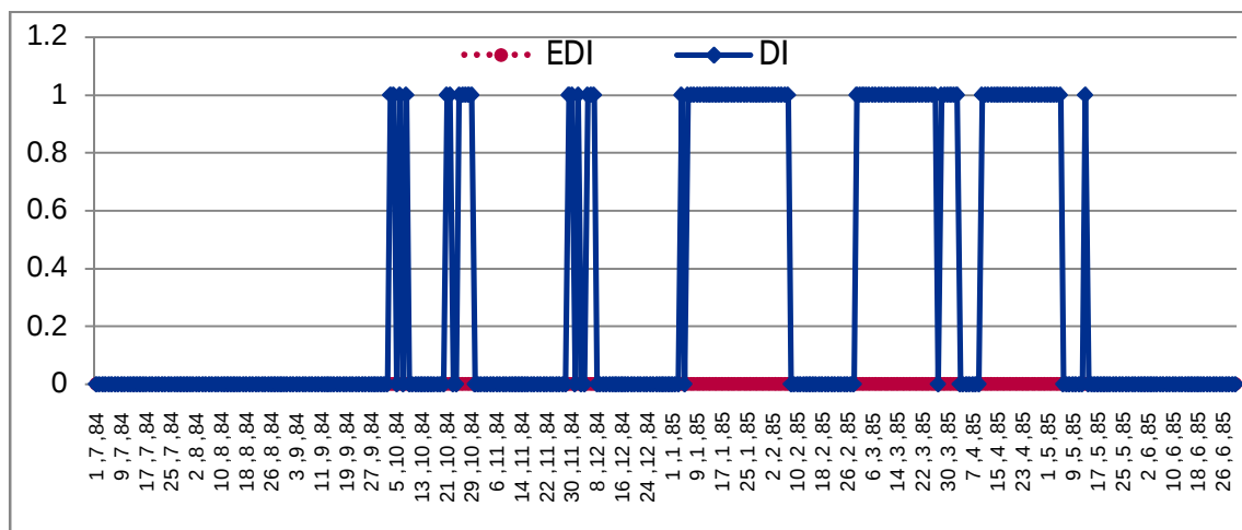
شکل 3-13: مقادیر شاخص‌های DI و EDI برای ایستگاه سسته طی سال‌های 1384 تا 1385 (1 و 0 به ترتیب وقوع و عدم وقوع خشکسالی را نشان می‌دهد)
