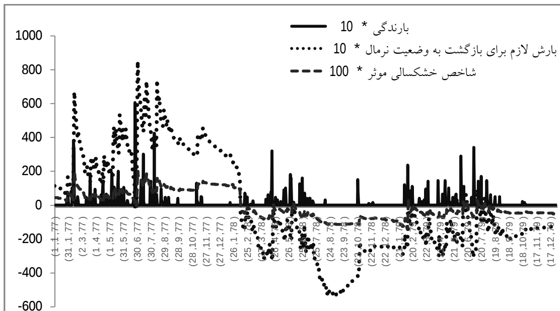
شکل 3-4: وضعیت روزانه خشکسالی طی سال آبی 1377-78 لغایت 1379-80
