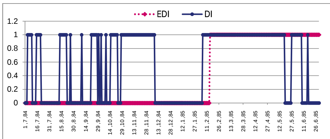
شکل 3-12: مقادیر شاخص‌های DI و EDI برای ایستگاه نقده طی سال‌های 1384 تا 1385 (1 و 0 به ترتیب وقوع و عدم وقوع خشکسالی را نشان می‌دهد)
