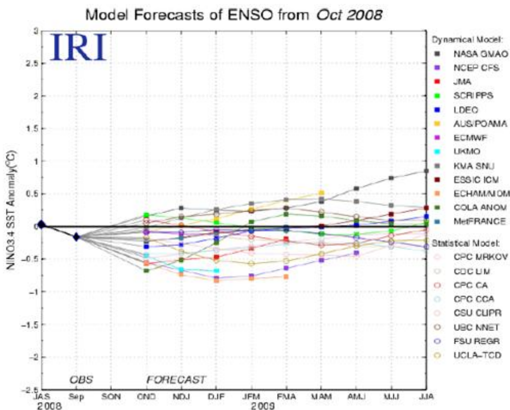
شکل 1-1: پیش‌بینی آنومالی دمای سطح دریا (SST) در منطقه NINO 3.4 (5°N-5°S, 120°W-170°W) توسط موسسه بین‌المللی تحقیقات اقلیم و جامعه (IRI)
