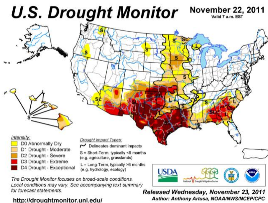
شکل 3-1: وضعیت خشکسالی در سطح آمریکا در تاریخ 2011/11/22
