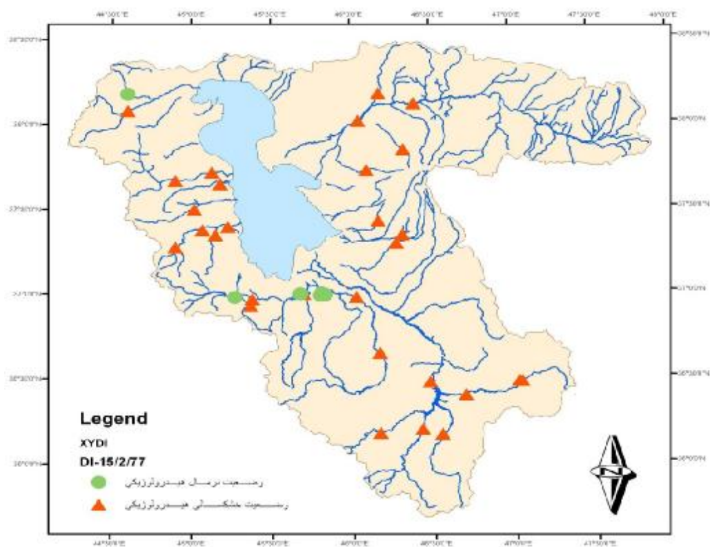
شکل 3-10: وضعیت هیدرولوژیکی خشکسالی در حوضه دریاچه ارومیه در تاریخ 1377/2/15
