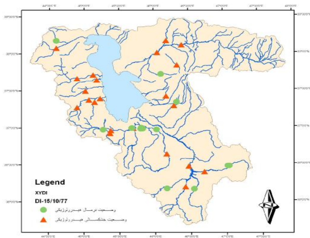
شکل 3-11: وضعیت هیدرولوژیکی خشکسالی در حوضه دریاچه ارومیه در تاریخ 1377/10/15
