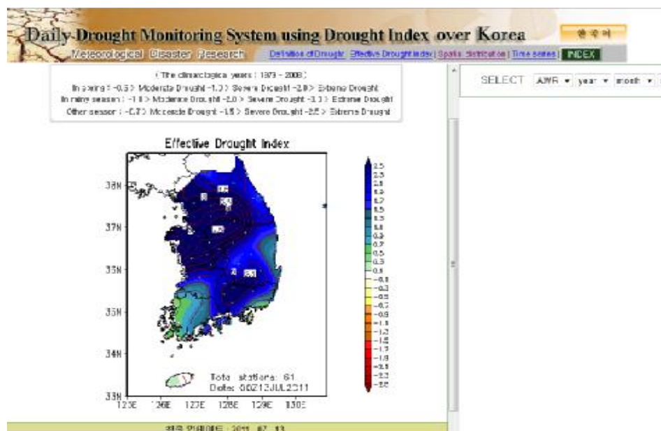
شکل 3-2: پایش روزانه خشکسالی در سطح کره جنوبی با استفاده از شاخص EDI برای 2011/7/13
