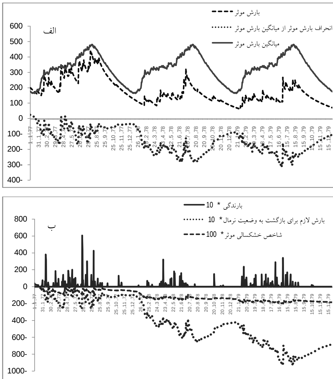
شکل 3-3: وضعیت روزانه خشکسالی EDI و سایر متغیرهای مربوط به این شاخص (میلی‌متر) طی سال آبی 1377-78 لغایت 1379-80 با استفاده از شاخص EDI در ایستگاه نقده
