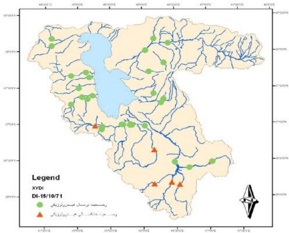
شکل 3-8: وضعیت هیدرولوژیکی خشکسالی در حوضه دریاچه ارومیه در تاریخ 1371/10/15
